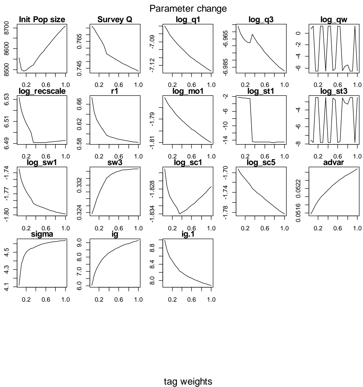
Figure B1-2. Changes in Parameter value.
